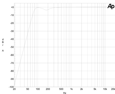
Amina AIWX EQ Response
